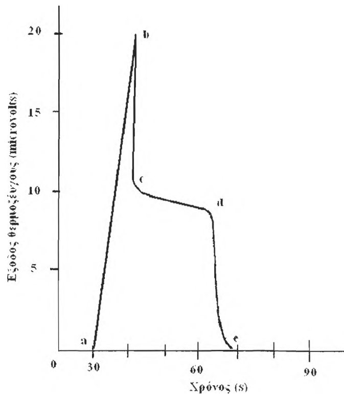
Εικόνα 13. Παραγωγή μικροτάσης ανά χρονικό διάστημα σε ψυχρομετρικό θερμοζεύγος εδάφους κατά την λειτουργία του. (Water in the environment, P. Rundel, W. Jarrell)
