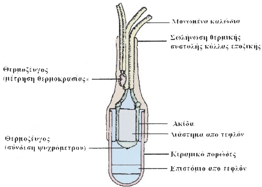
Εικόνα 12. Δομή ενός τυπικού ψυχρόμετρου εδάφους. (Water in the environment, P. Rundel, W. Jarrell)
