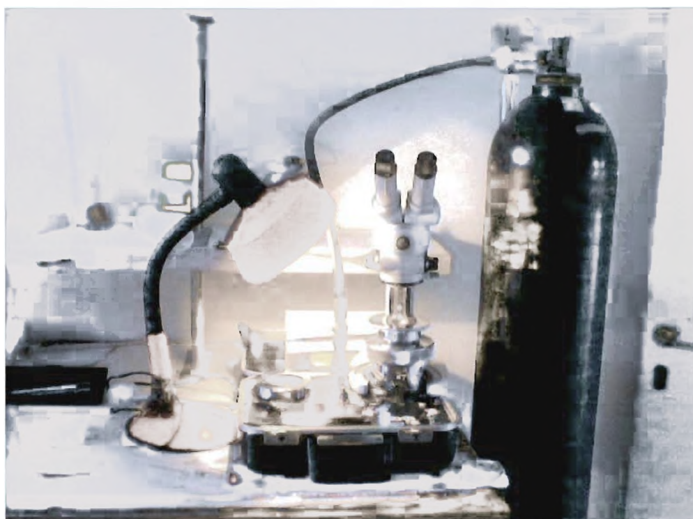
Εικόνα 37. Διάταξη ενός οργάνου πιεστικού θαλάμου. (Από το πείραμα που πραγματοποιήσα)
