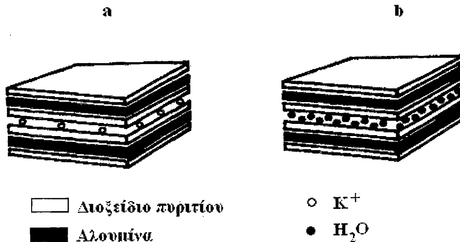
Εικόνα 9. Διάταξη στρώματος διοξειδίου του πυριτίου και αλουμίνας σε (a) αδιατάρακτο ιλλίτη και (b) διογκούμενο μοντμοριλλονίτη. (Water stress on plants, G. M. Simpson)
