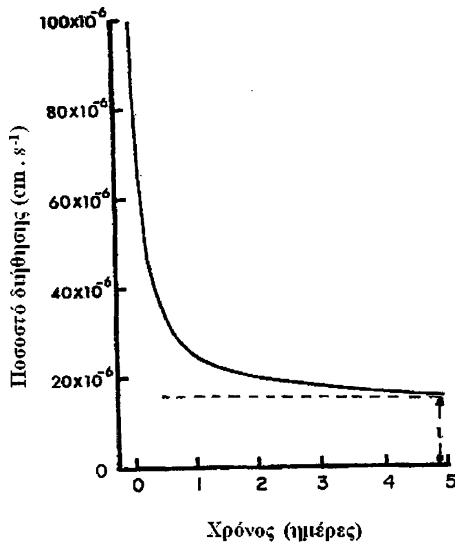
Εικόνα 4. Ρυθμός διήθησης νερού στο έδαφος σε χρονικό διάστημα. (Water stress on plants, (G. M. Simpson)
