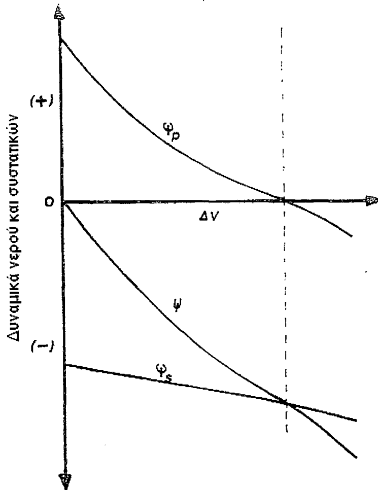
Εικόνα 31. Σχέση μεταξύ του όγκου της απώλειας νερού ( \Delta V ) του νερού ( \psi ) και των συνιστωσών δυναμικών του, της διαλυτής ουσίας ( \Psi_s ), και δυναμικό πίεσης ( \Psi_p ), σε κύτταρο που παρουσιάζει ιδανική οσμωτική συμπεριφορά. (Water stress on plants, G. M. Simpson)
