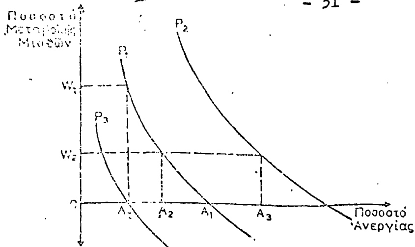
Διάγραμμα 17.8. Η καμπύλη τού Phillips
