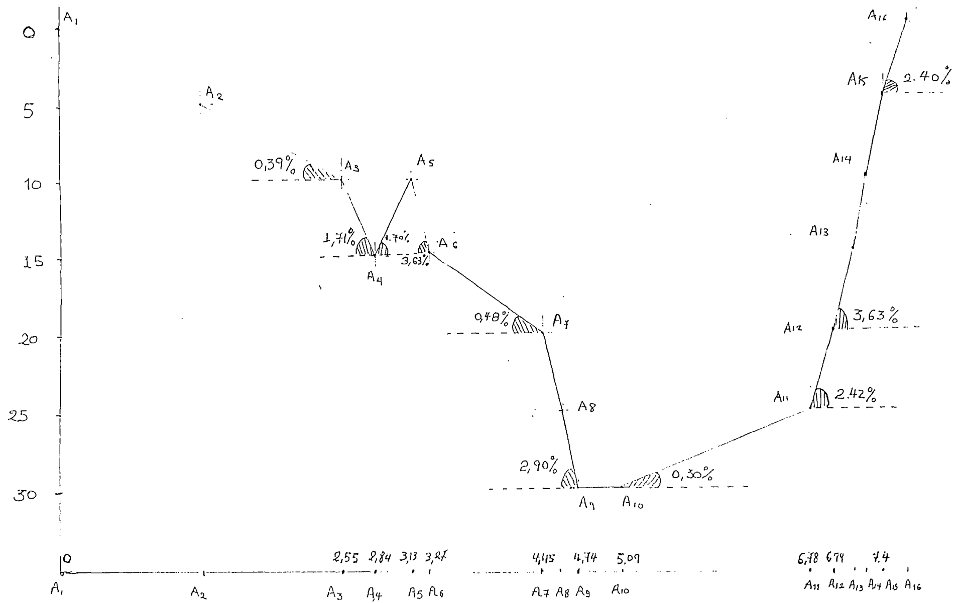
Σχήμα 4.3 - Τομή κατά τον άξονα ΑΑ με τις κυριότερες κλίσεις του πυθμένα.
