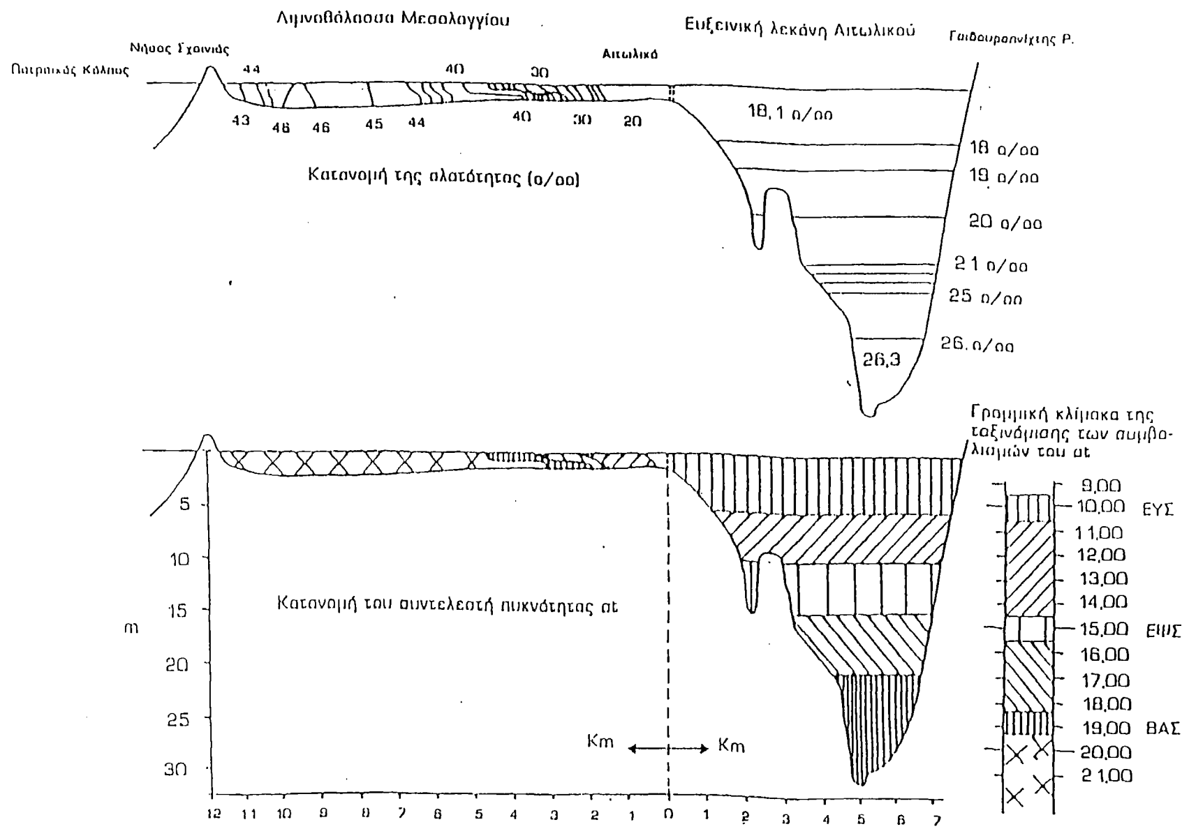
Σχήμα 4.6 Κατανομή της αλατότητας (επάνω) και της πυκνότητας (κάτω) με το βάθος σε μια μορφολογική τομή διεύθυνσης Ν-Β-ΒΔ κατά μήκος της Λιμνοθάλασσας Μεσολογγίου και της λεκάνης Αιτωλικού. Διακρίνεται η στρωμάτωση των διαφόρων τύπων νερού της περιοχής.
